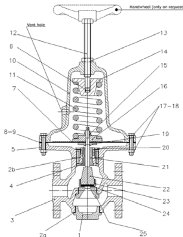
R620 系列阀门剖面图
