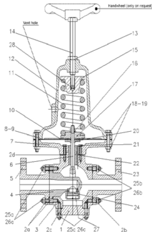
R610 系列阀门剖面图
