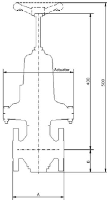
法兰连接剖面图
