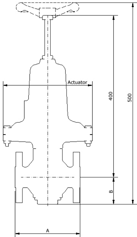
法兰连接剖面图
