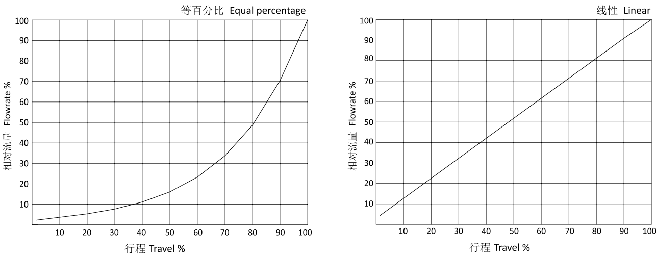
波纹管控制阀流量特性曲线（等百分比、线性） Bellows valve flow characteristic flow chart(Equal percentage/Linear)
